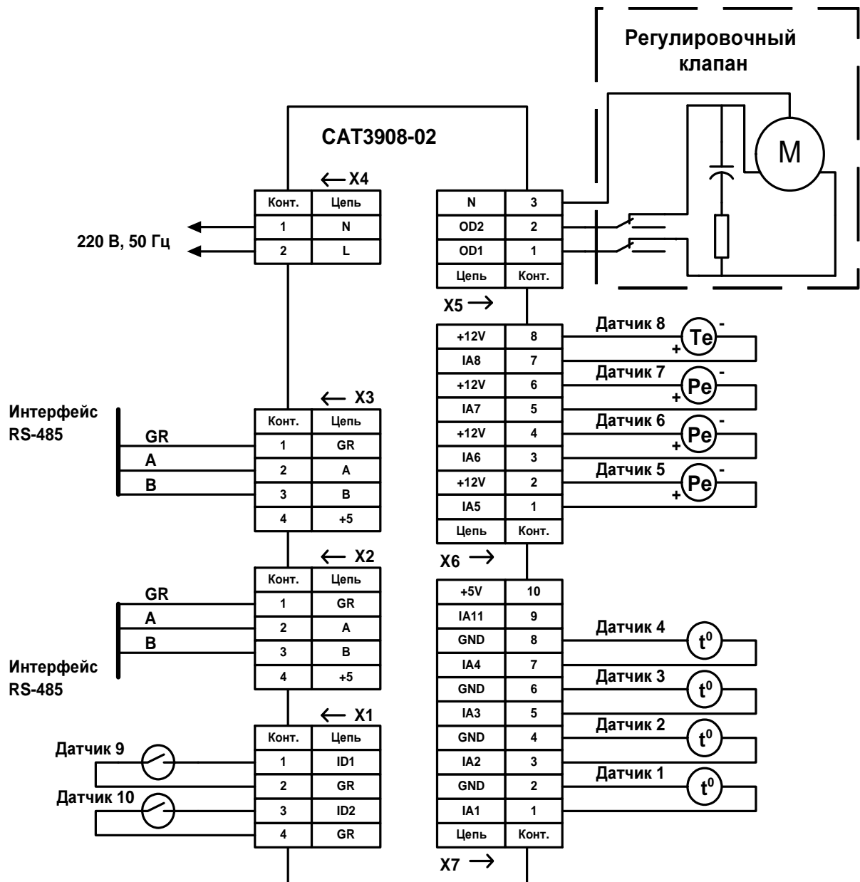
Рисунок 6 - Электрическая принципиальная схема подключения САТ3908-02 (типовая)
