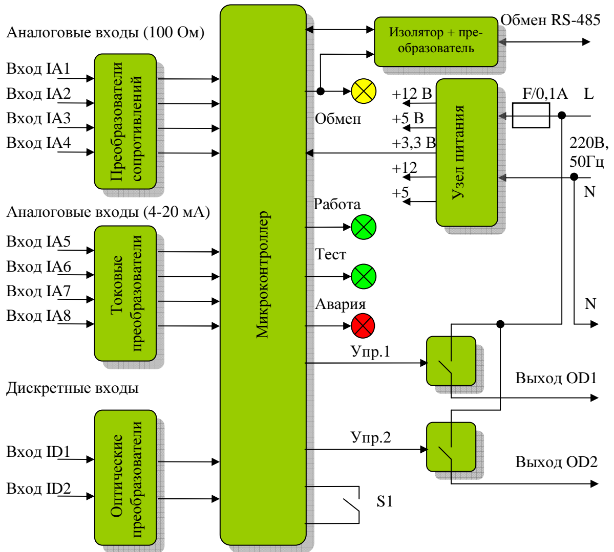
Рисунок 3 - Структурная схема САТ3908-02
