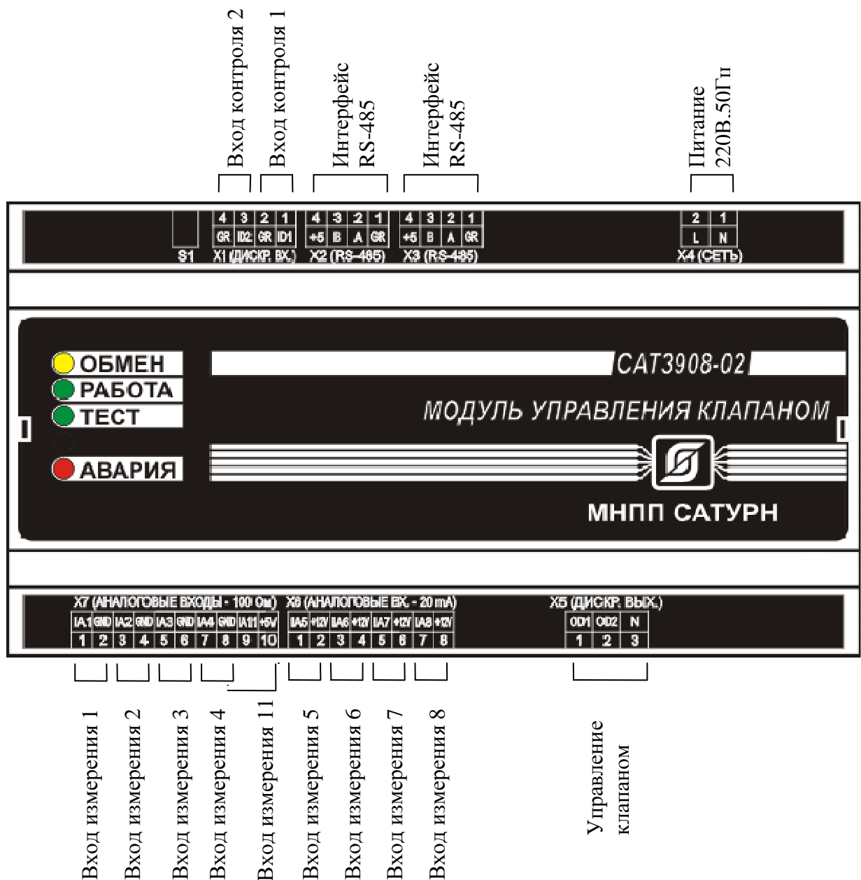
Рисунок 5 - Расположение разъёмов на модуле CAT3908-02
